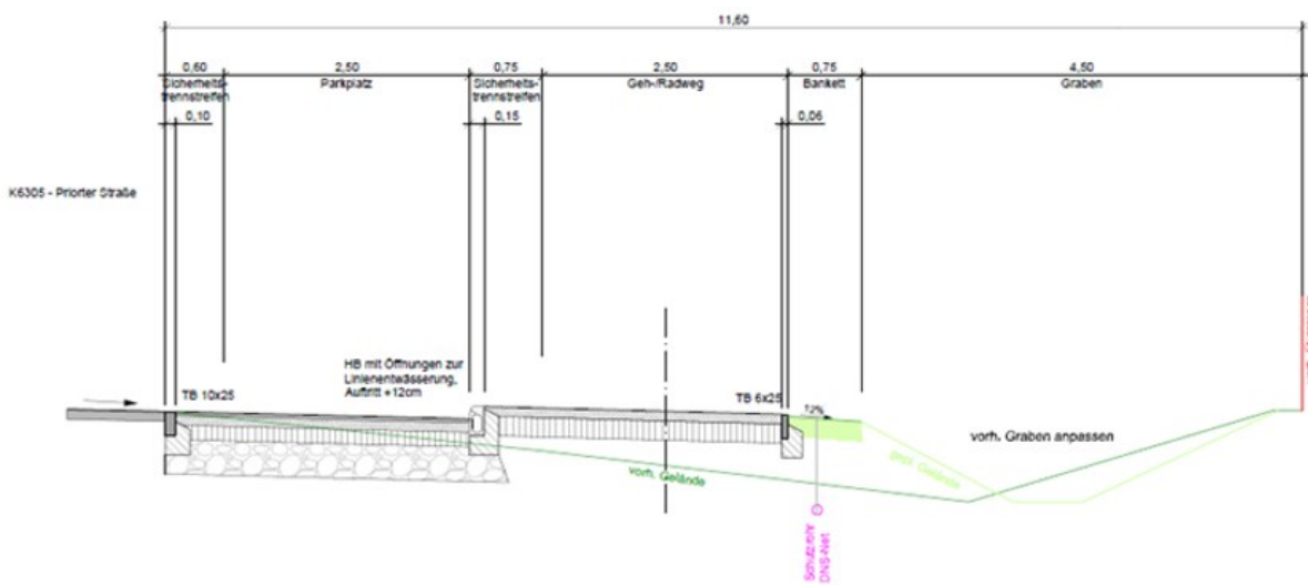
Abbildung 4 Querschnitt der Park- und Radwegflächen
