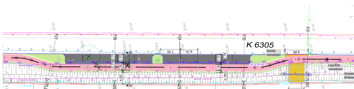
Abbildung 3 Draufsicht der geplanten Maßnahme
