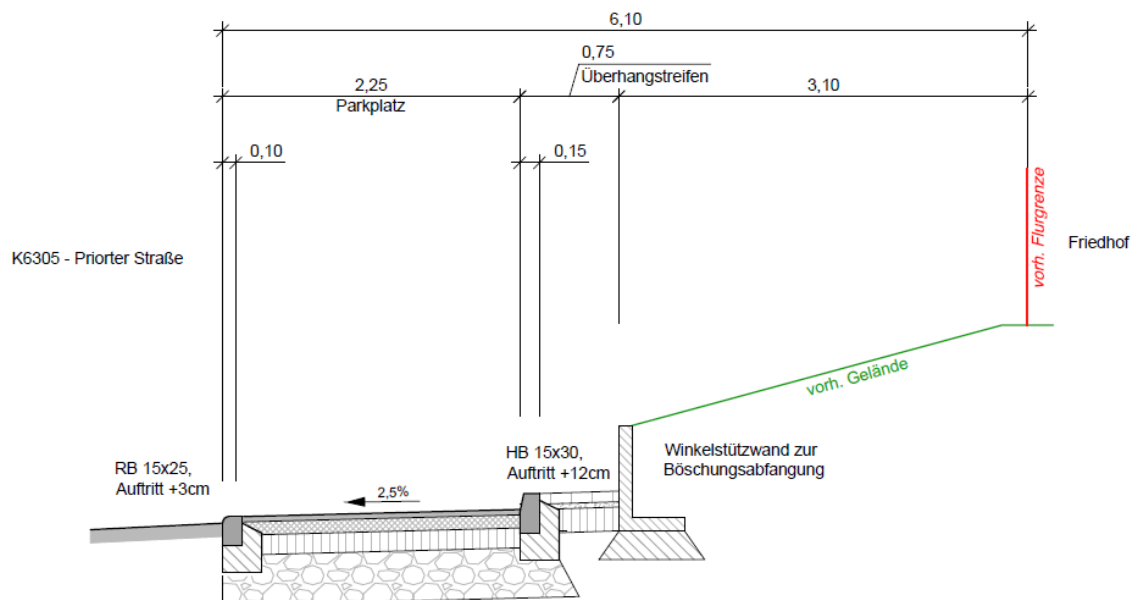
Abbildung 2 Querschnitt der Längsparker am Friedhof
