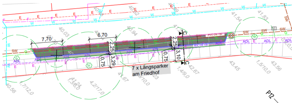
Abbildung 1 Draufsicht der Längsparker am Friedhof
