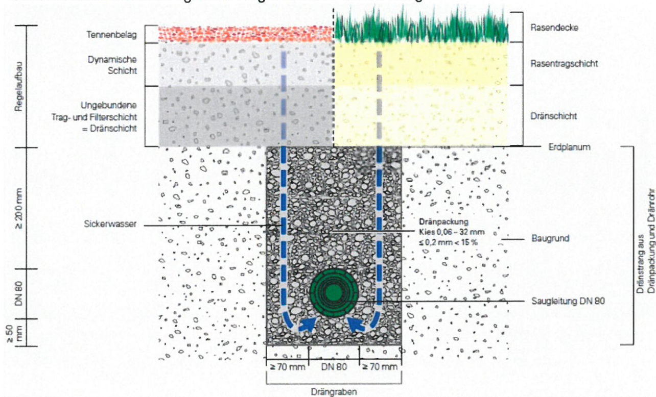
Schematische Darstellung eines Regelaufbaus mit Dränung
