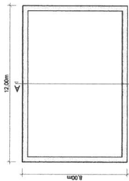
Grundriss _ Wohnhaus 2
