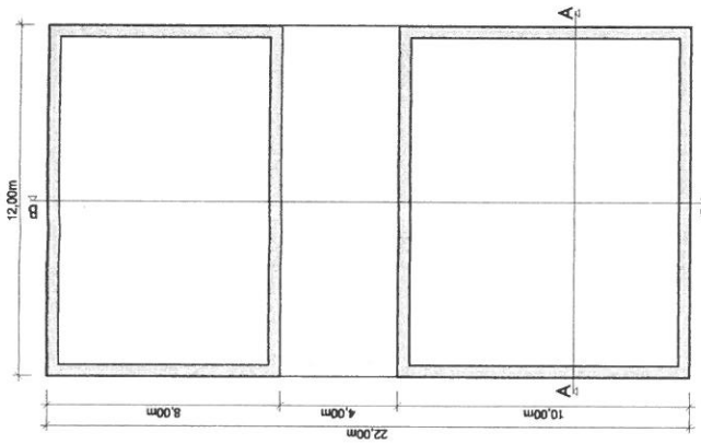
Grundriss _ Wohnhaus 3
