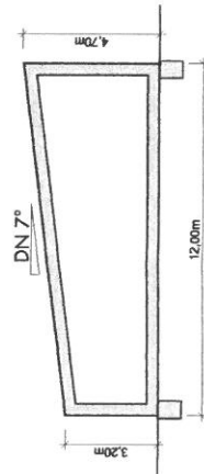
Schnitt A _ Wohnhaus 3
