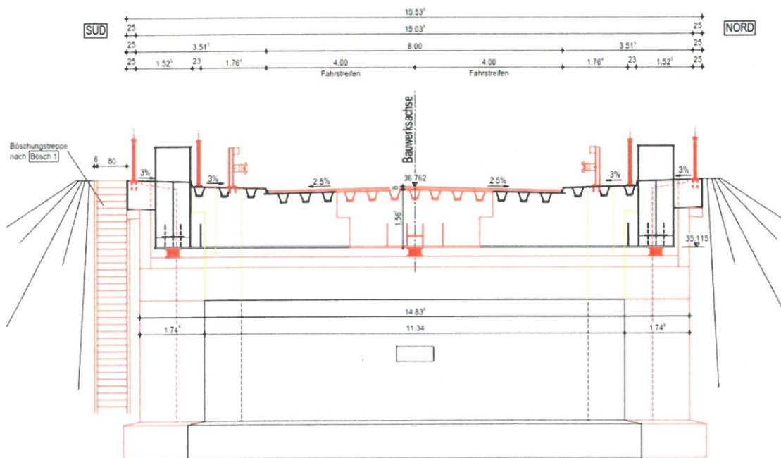
Widerlageransicht Achse 20
