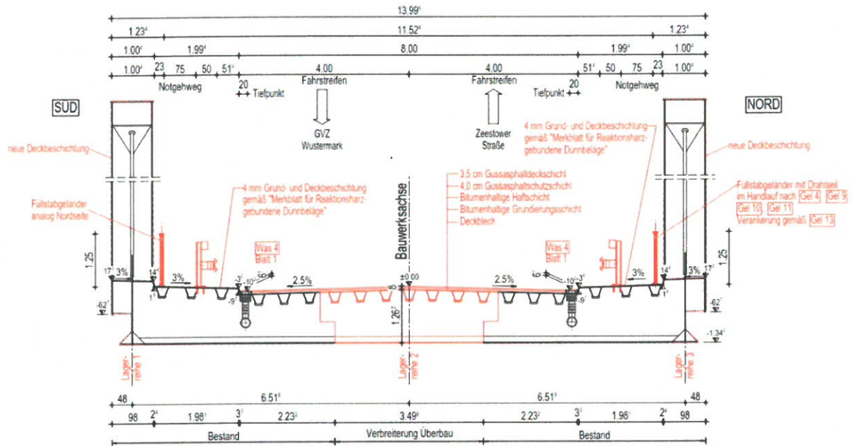
Regelquerschnitt M. 1:50
