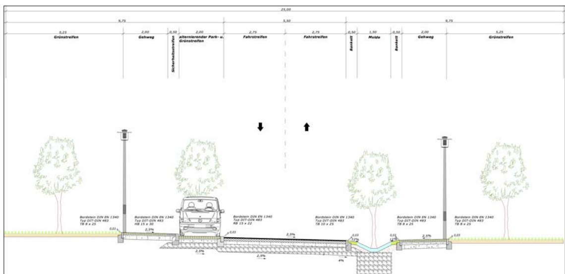
Abb.: Prinzipquerschnitt der Planstraße B (mittlerer Bereich) (25 m)
