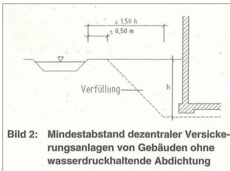
Abb.: Schema des Sicherheitsabstandes, Auszug aus ATV-DVWK-A 138
