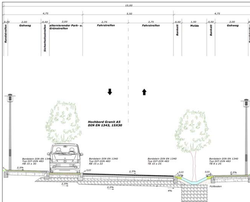
Abb.: Prinzipquerschnitt der Planstraße B (15 m)
