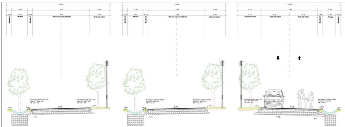
Abb.: Prinzipquerschnitte der Planstraße A und C (links), D (mitte) und E (rechts)
