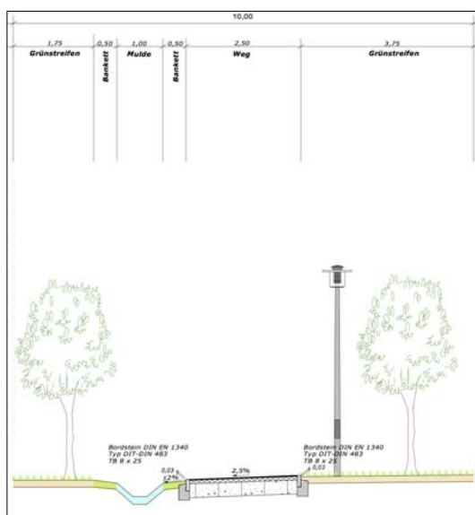
Abb.: Prinzipquerschnitt des Weges
